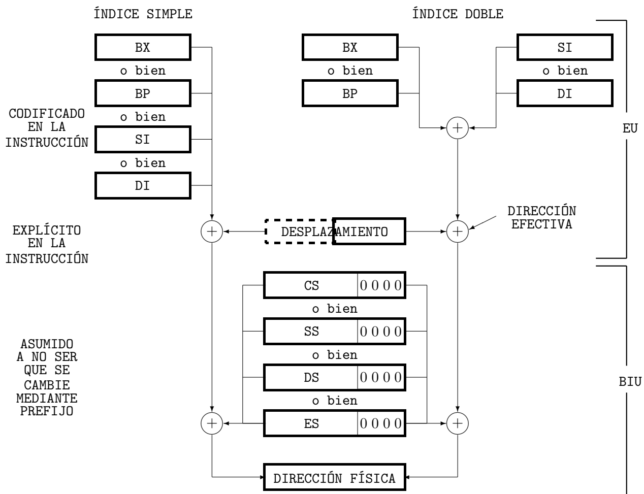
Cálculo de la dirección de memoria en el procesador Intel 8086
