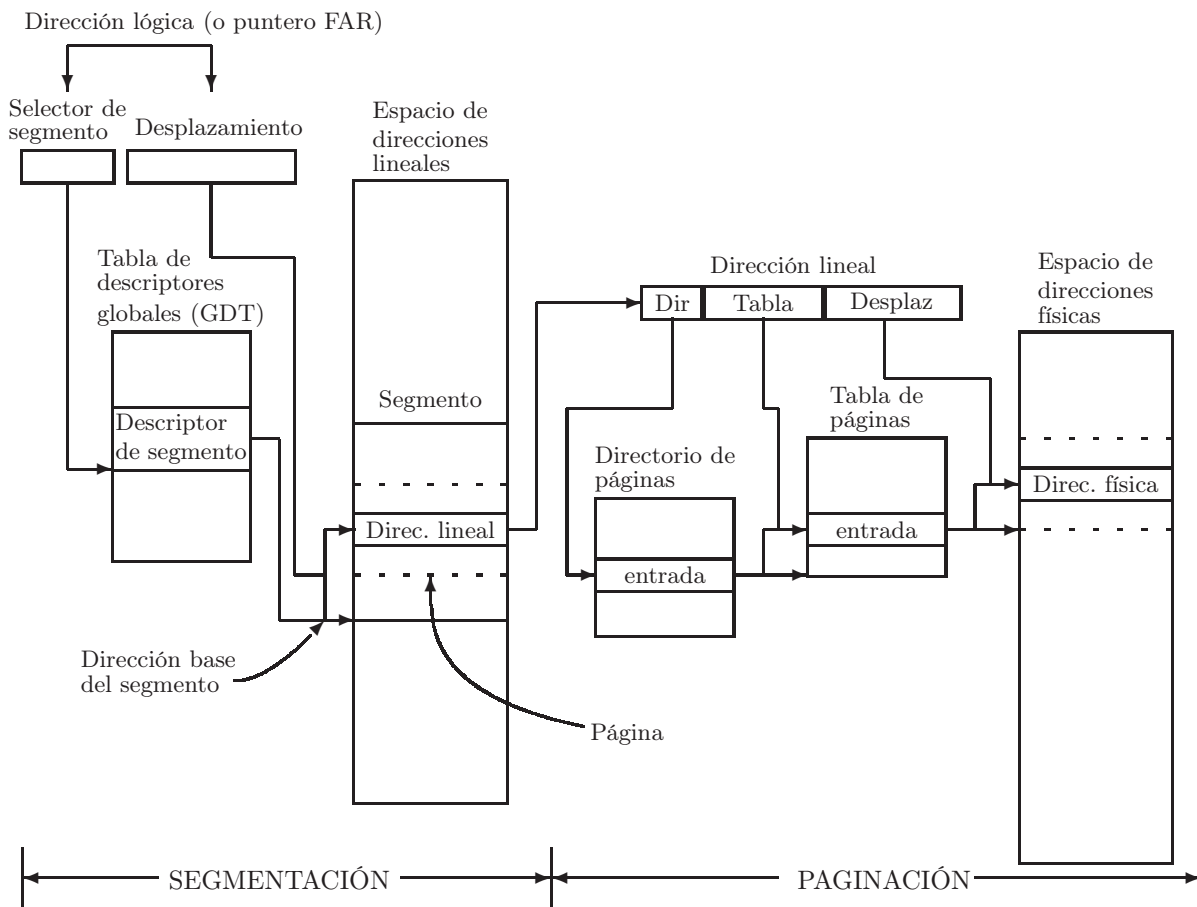
Segmentación y paginación en la IA-32
