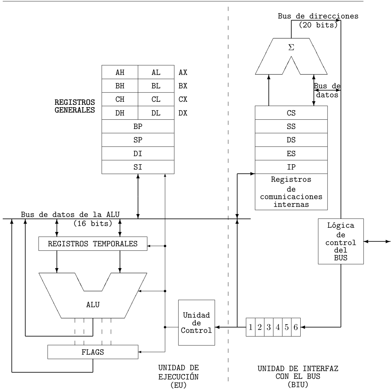
Estructura del procesador Intel 8086
